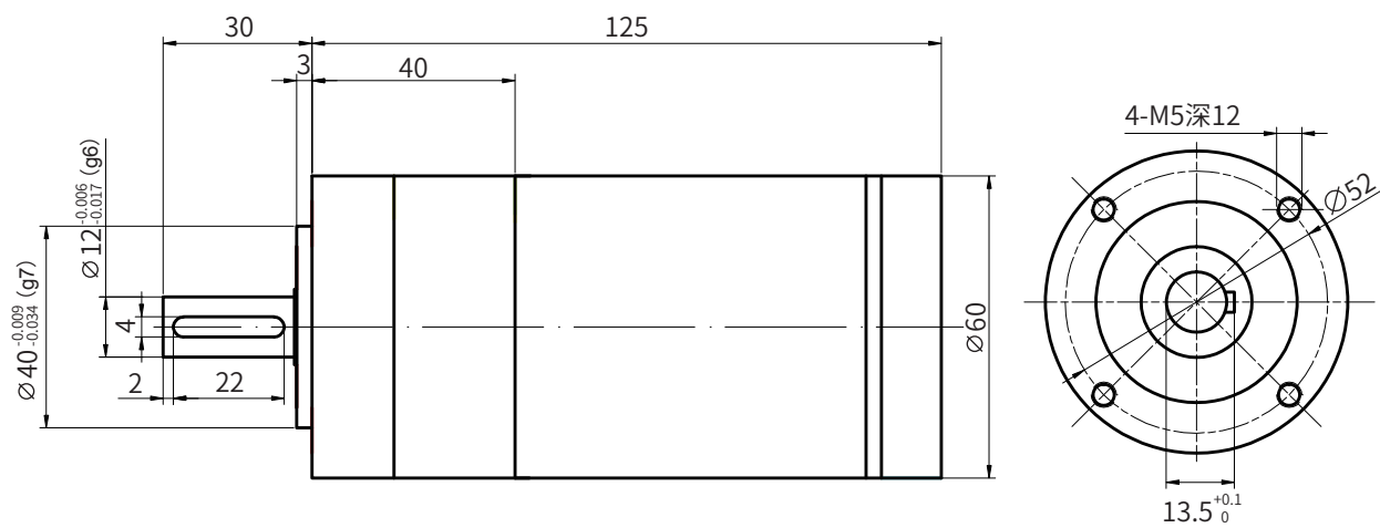
减速机输出端安装尺寸
