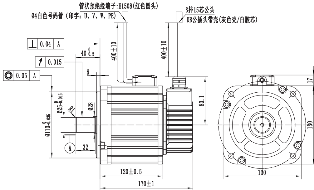
电机尺寸图（单位:mm）
