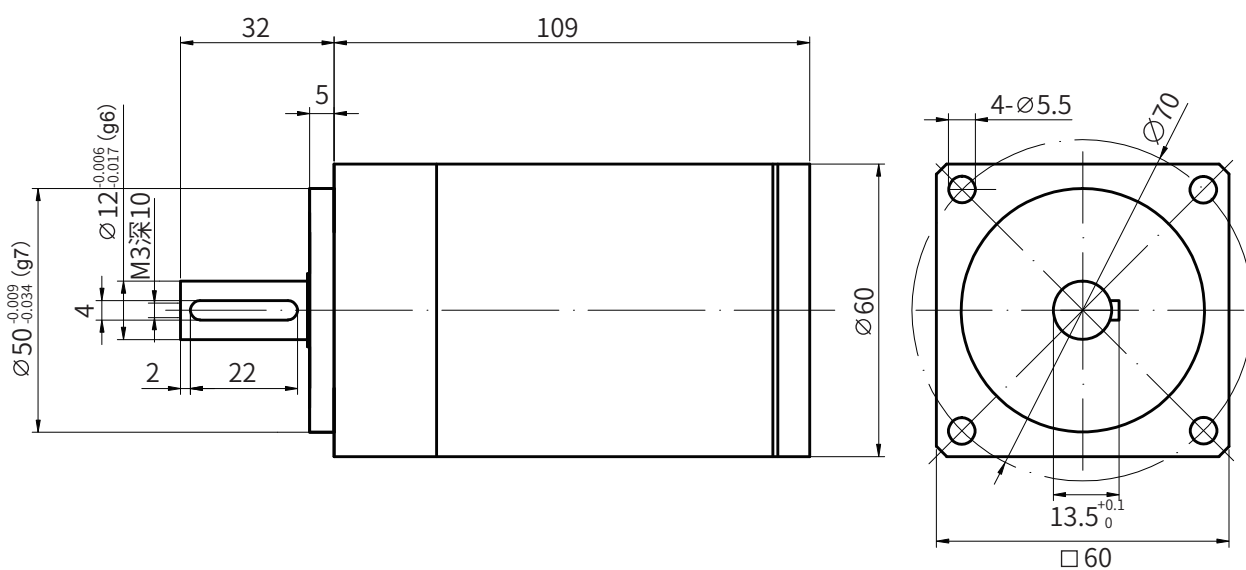
减速机输出端安装尺寸
